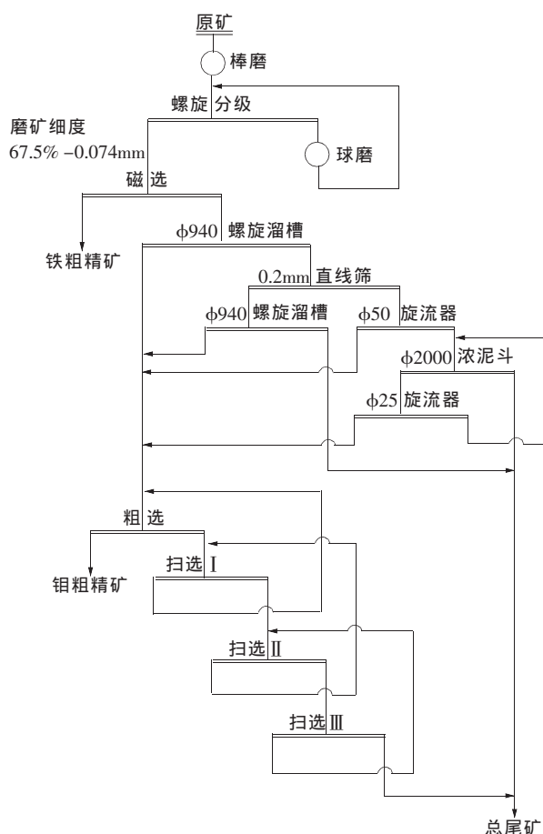
图 1 半工业试验流程
