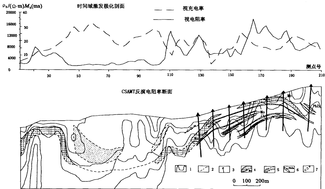
图 3 小东沟钼矿 50 线地质物探综合剖面图
