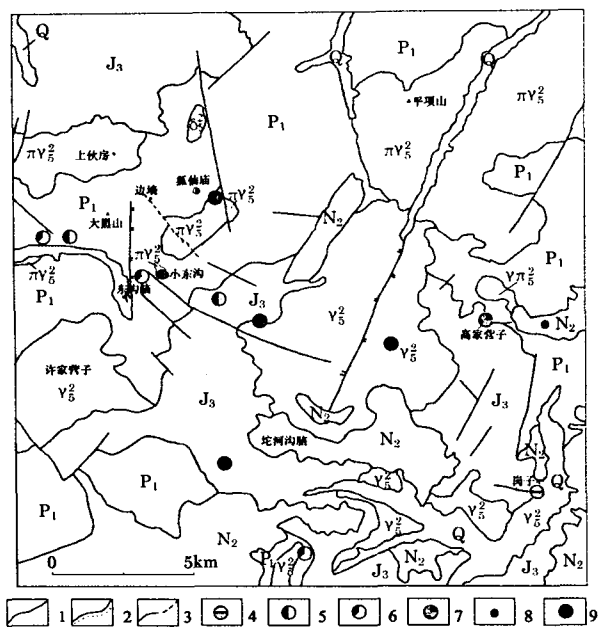
图2 小东沟钼矿区域地质示意图
