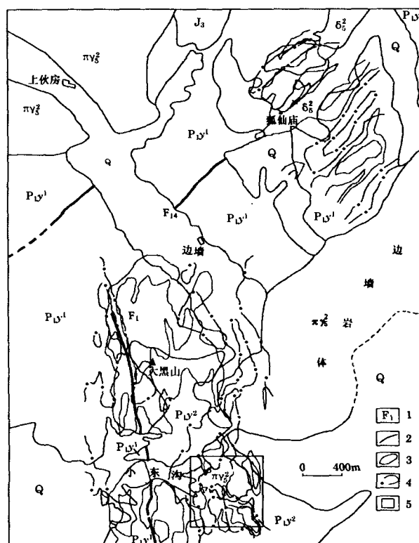
图1 小东沟地区综合地质图
