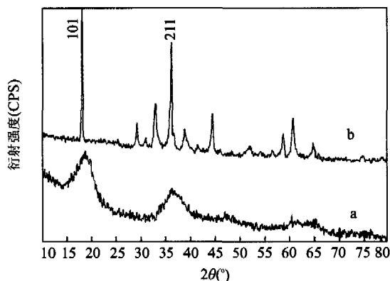
图 4 微波烧结前(a)和微波烧结后(b)样品的 XRD 图
