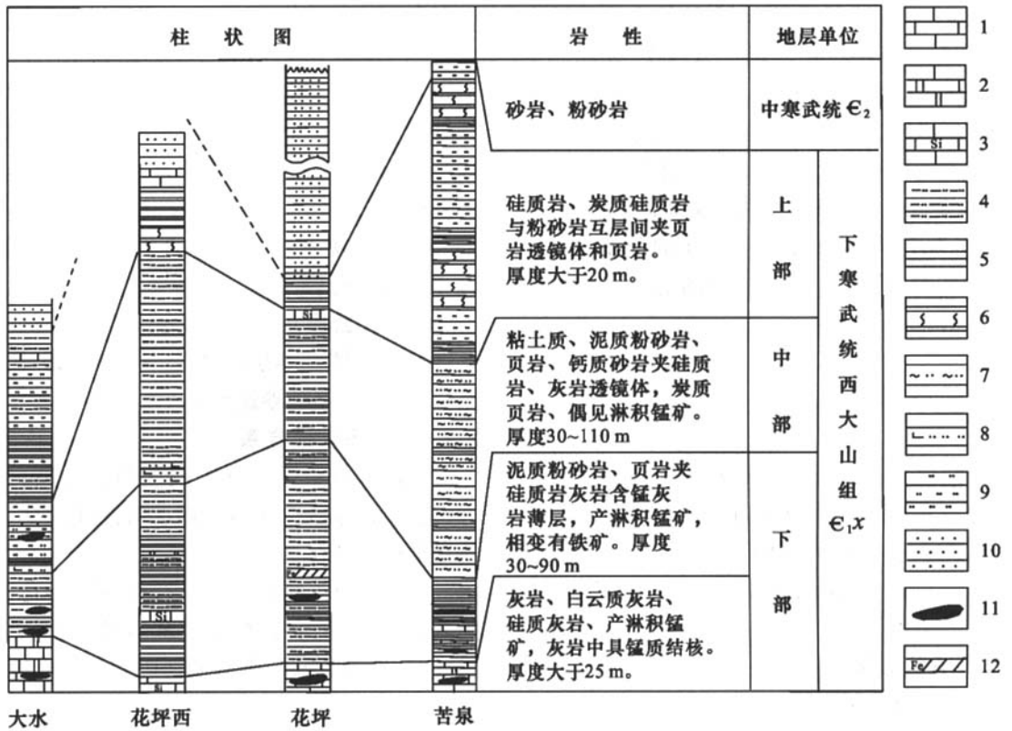
图2 大水、花坪、苦泉锰矿区中、下寒武统地层柱状图
